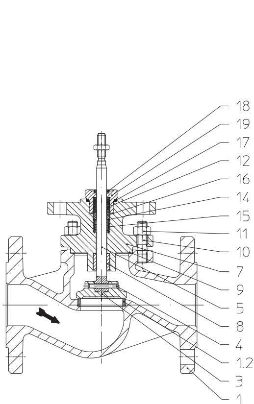
Bild 1: BR 405 Standardausführung
