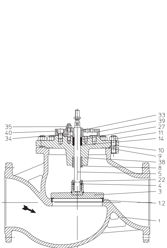
Bild 3: BR 405 DN125v-150v / DN200-250
