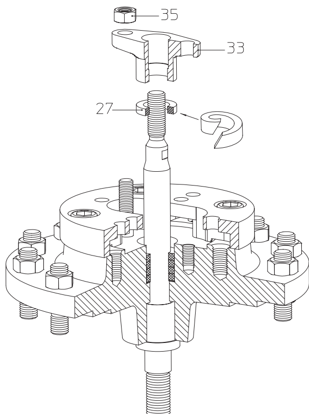
Bild 15: Stopfbuchspackung DN125v-150v / DN200-250
