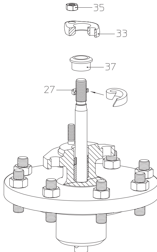
Bild 14: Stopfbuchspackung DN125-150
