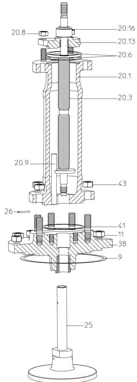
Bild 18: BR460 DN125v-150v / DN200-250
