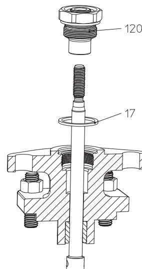
Bild 10: EPDM Abdichtung DN15 – DN100
