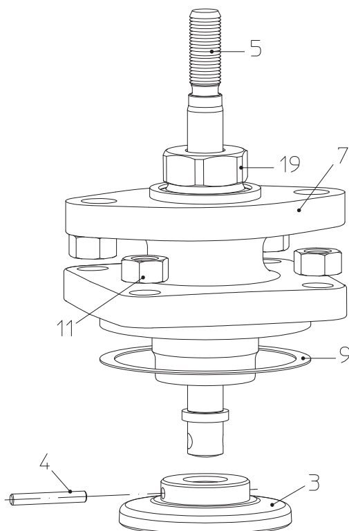
Bild 19: BR405 DN15-100
