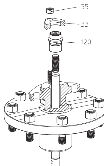
Bild 11: EPDM Abdichtung DN125 – DN150
