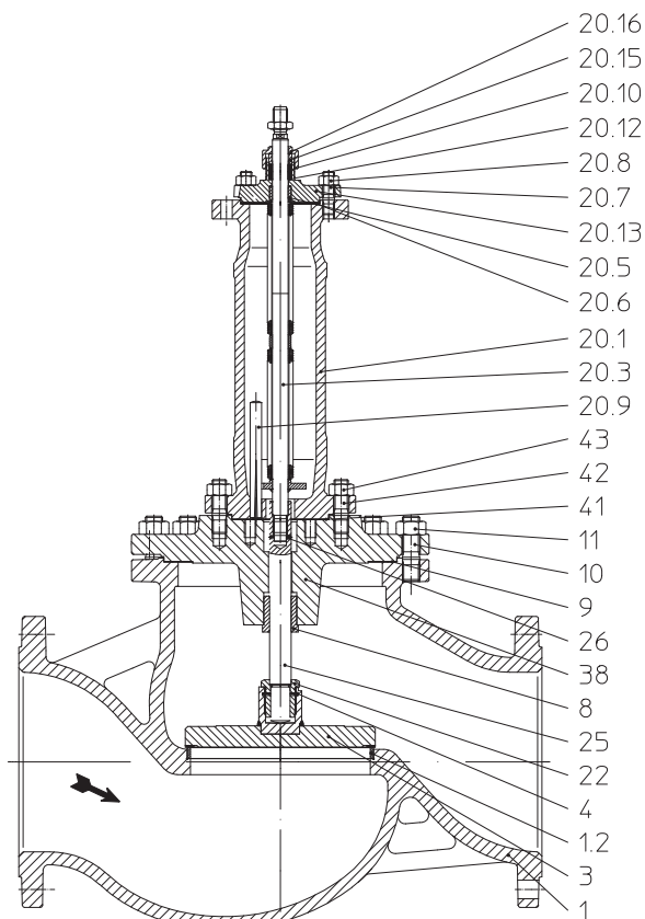
Bild 4: BR 460 DN125v-150v / DN200-250
