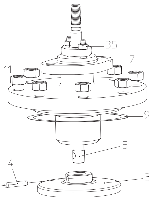
Bild 20: BR405 DN125-150
