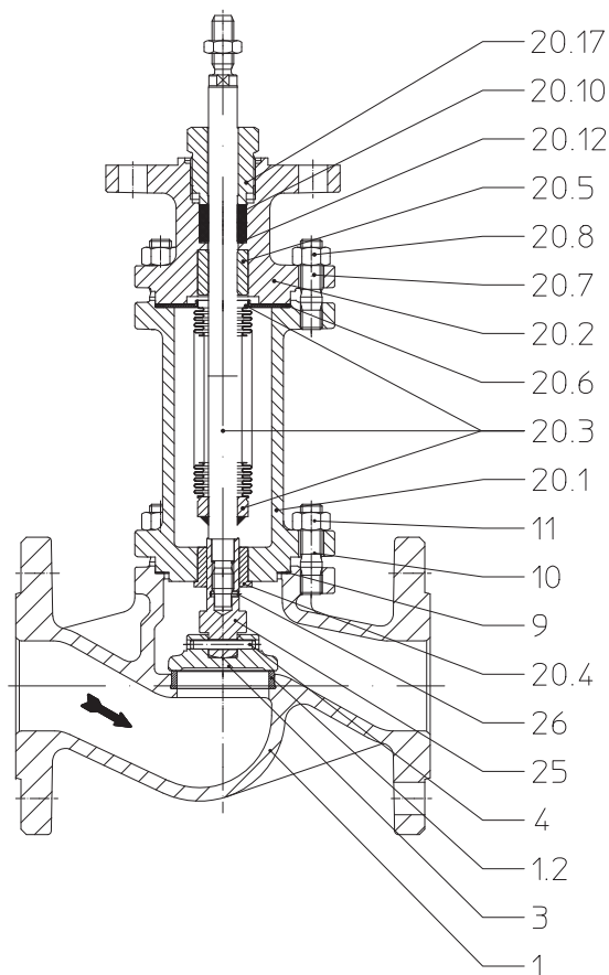
Bild 2: BR 460 Standardausführung
