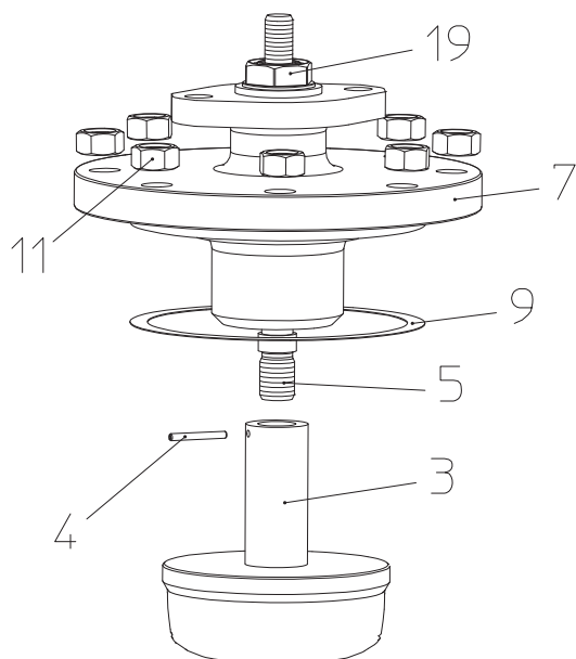
Рис. 25: BR 440 / 445 DN125-150
