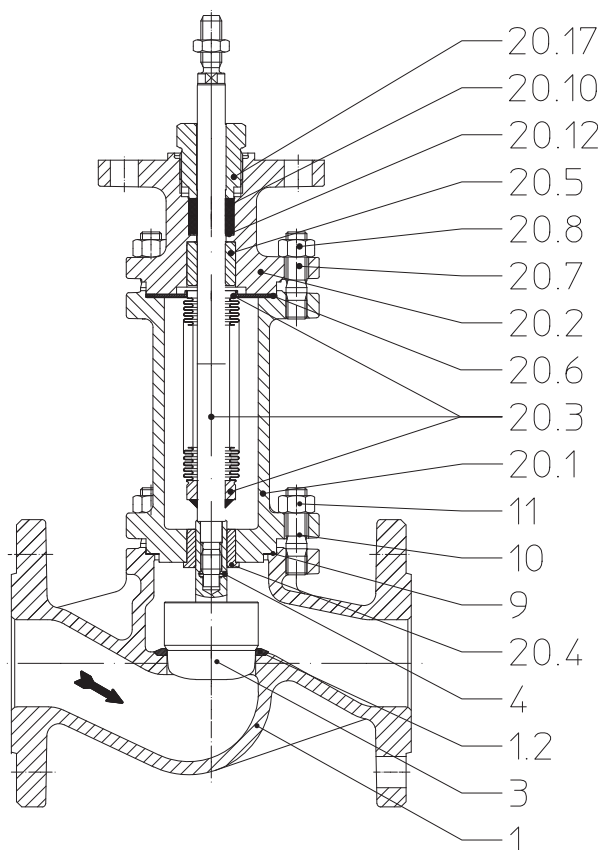
Рис. 2: BR 441 DN15-100
