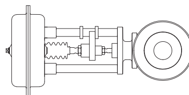
Рис. 17: горизонтальный трубопровод
