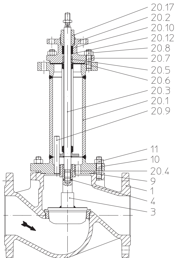
Рис. 10: BR 446 DN125-150 (только нержавеющая сталь)
