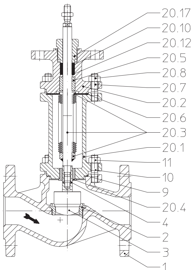
Рис. 8: BR 446 DN15-100 (только нержавеющая сталь)
