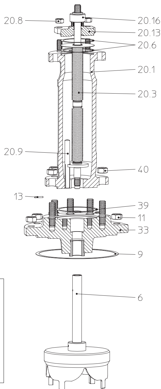
Рис. 23: BR 441 DN200-250
