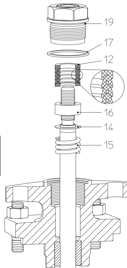
Рис. 18: Шевронное кольцо DN15-150
