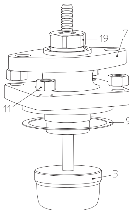
Рис. 24: BR 440 / 445 DN15-100
