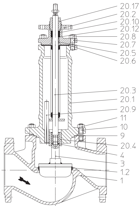
Рис. 4: BR 441 DN125-150
