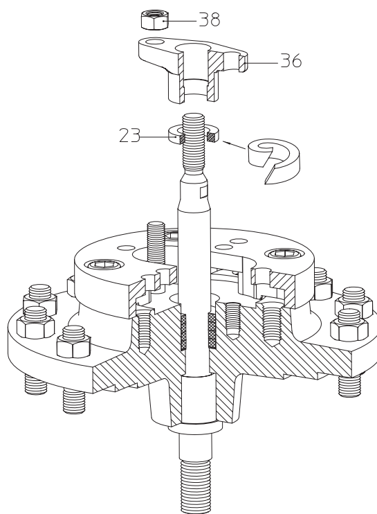
Рис. 20: сальниковая набивка DN125v-150v / DN200-250
