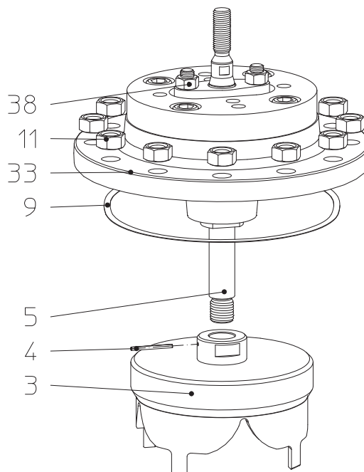
Рис. 26: BR 440 / 445 DN200-250
