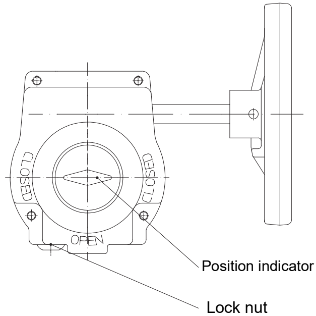
Fig. 4: Worm gear
