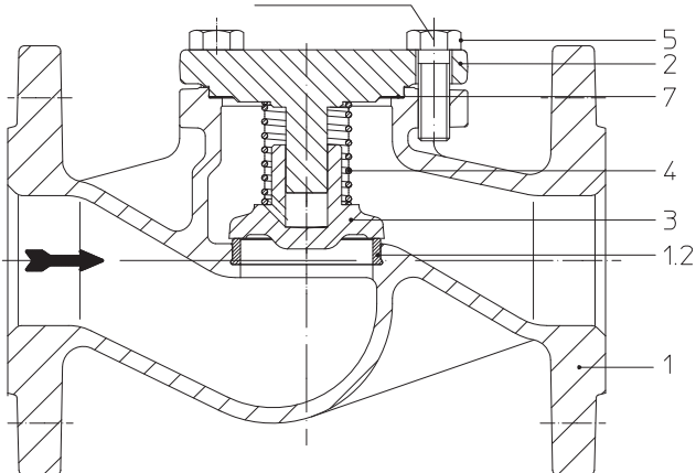
Рис. 3: CHECKO®-V - DG PN6-16 EN-JL1040
