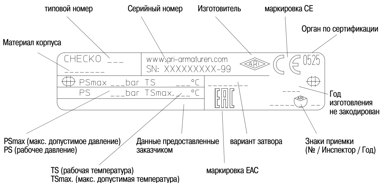
Рис. 8: Типовая табличка (шилдь)
