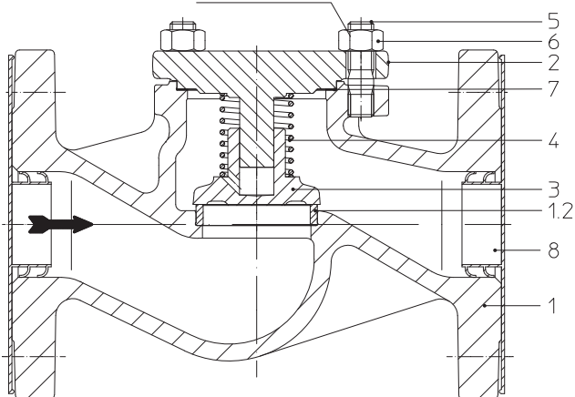
Рис. 1: CHECKO®-V - DG PN16-40 EN-JS1049 / 1.0619+N
