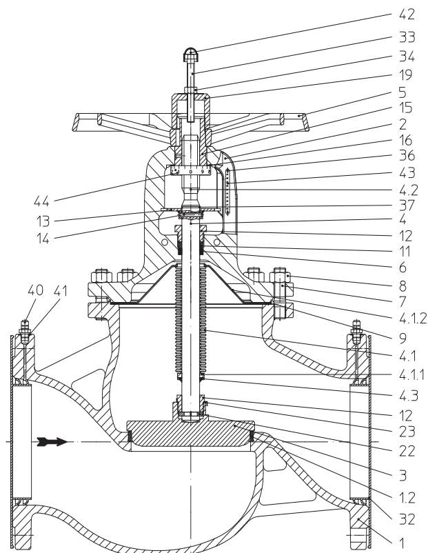
Bild 4: DN 200 mit Hubskala
