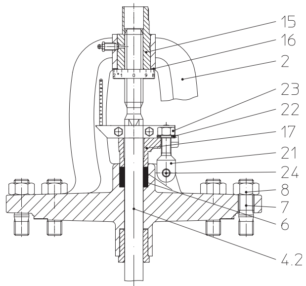
Bild 8: DN250-400
