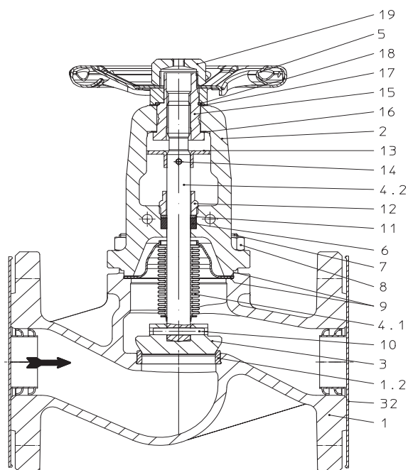
Рис. 1: FABA®-Plus - проходная конструкция
