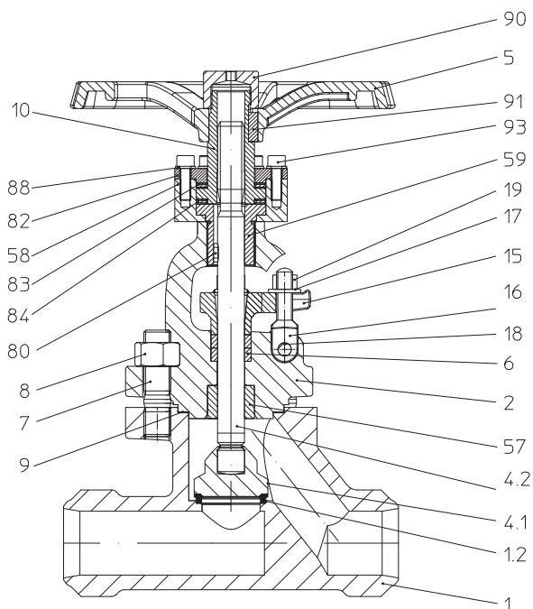
Рис. 6: STOBU проходная конструкция, фланцевое соединение, соединение концы под приварку DN 10-50 с неподнимающимся маховиком
