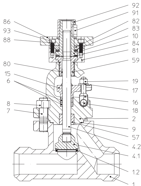
Рис. 8: STOBU проходная конструкция, фланцевое соединение DN 10-50 с соединением ISO 5210 группа (фланцевый переходник) B1
