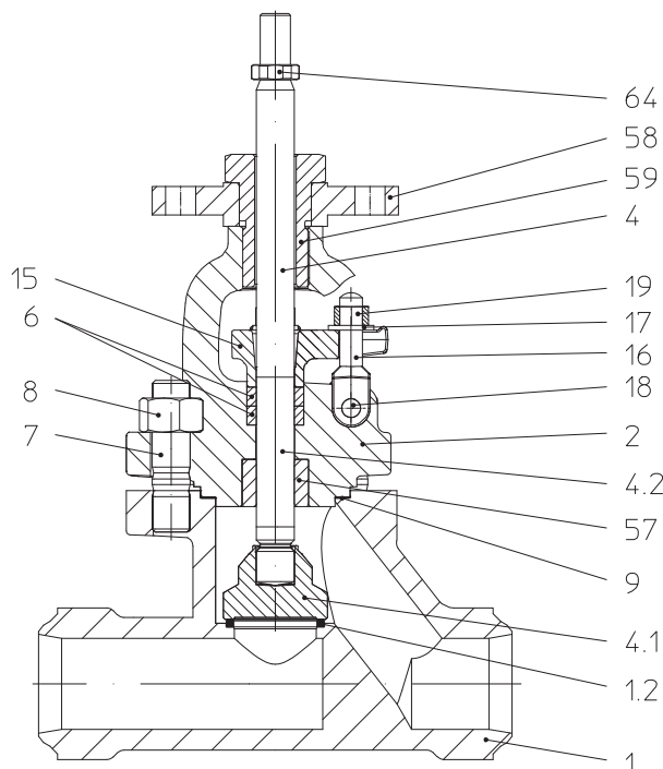
Рис. 7: STOBU проходная конструкция, фланцевое соединение DN 10-50 с соединением ISO 5210 группа A
