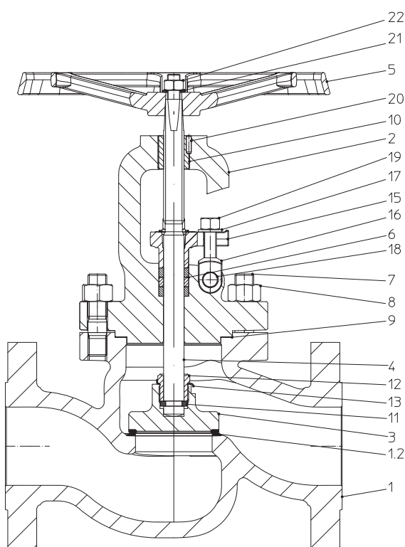
Рис. 3: STOBU проходная конструкция, фланцевое соединение DN 65-100
