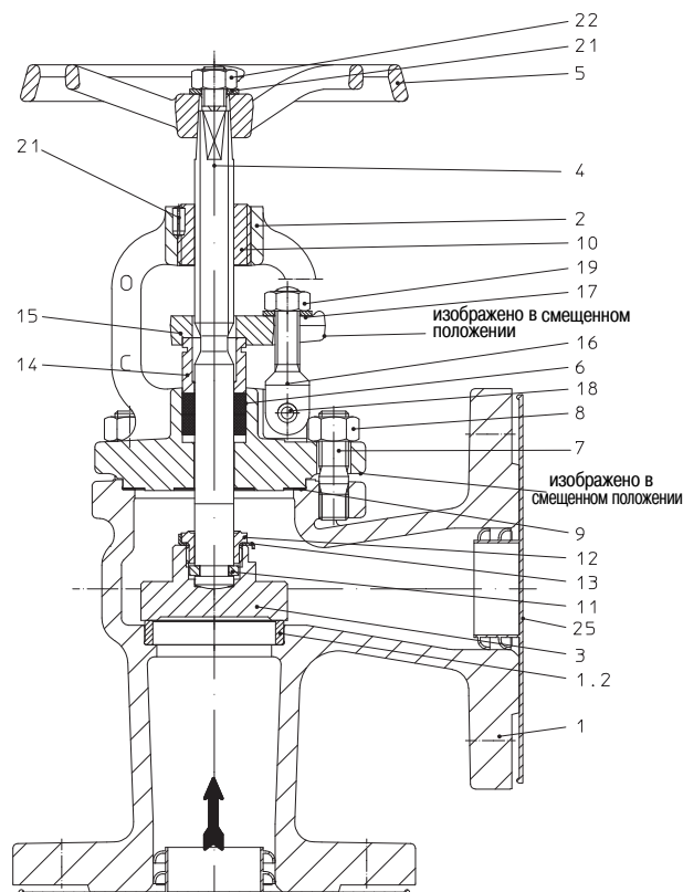
Рис. 2: STOBU-ECK 1.0619+N
