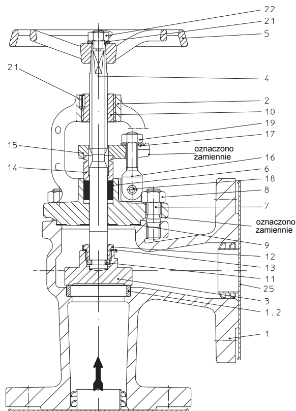
Rys. 2: STOBU-ECK 1.0619+N
