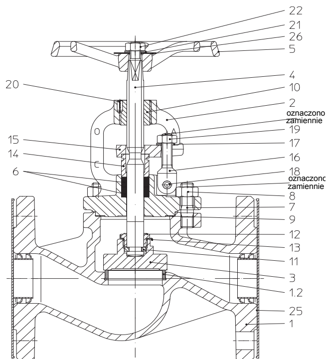
Rys. 1: STOBU-DG 1.0619+N
