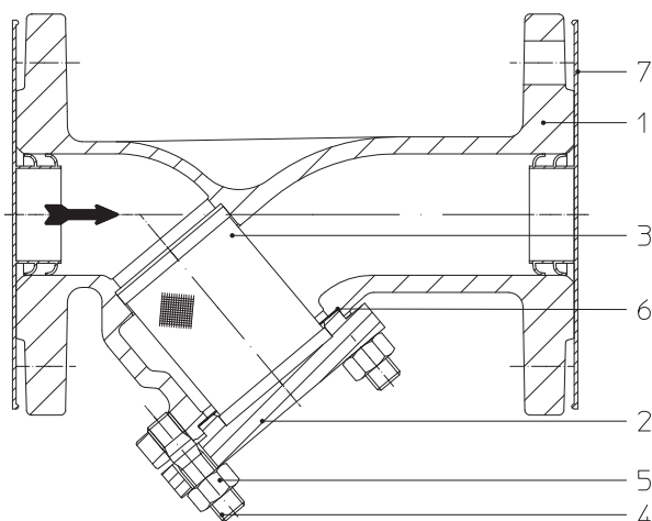
Рис. 1: Грязеуловитель - Y
