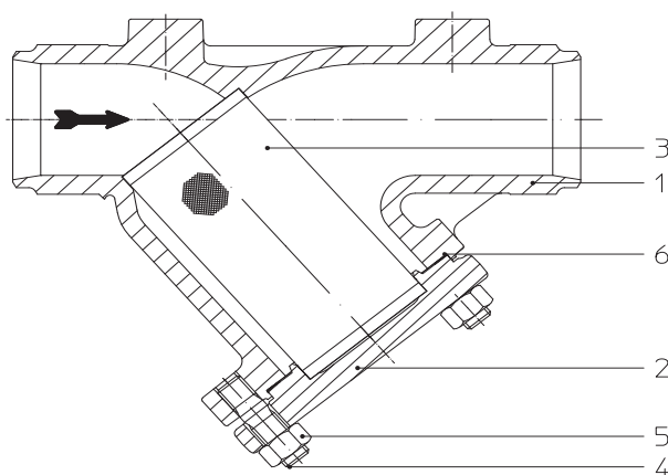
Рис. 2: Грязеуловитель - Y SE
