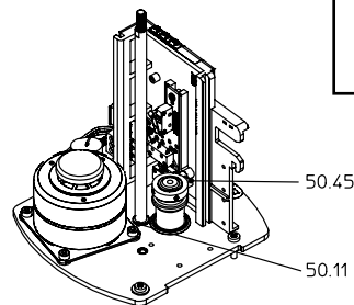
BLDC-мотор 24В AC/DC
