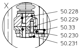
Coupling 25 kN
